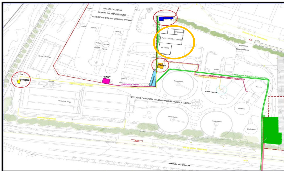
Plànol 1. Planta de tractament tèrmic eficient de Mataró. Planta General d'edificis i elements
