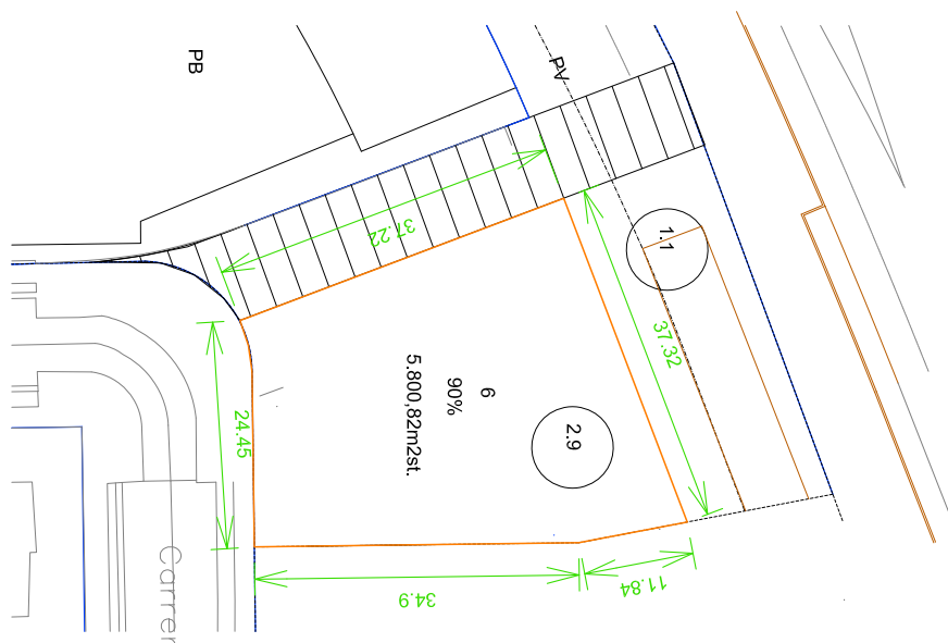
REPLANTEIG E: 1/500
